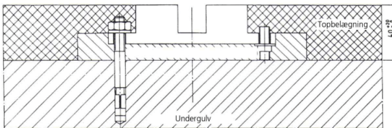
Styreskinne
