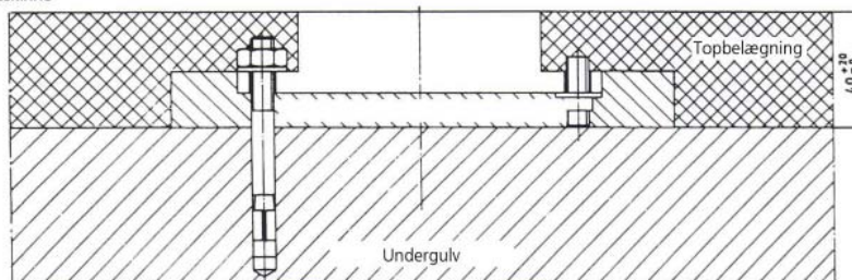
Løbeskinne
